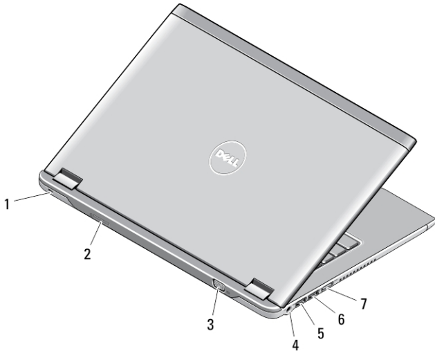
Abbildung 2. Rückansicht
